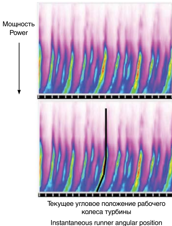
Рис. 6: Различные участки – следы взаимодействия различных пар направляющих/рабочих лопаток
